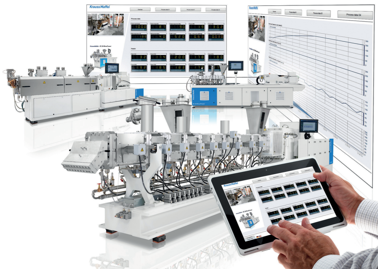
整个克劳斯玛菲ZE BluePower双螺杆挤出机- 完美地为智能工厂解决方案做好了准备。
